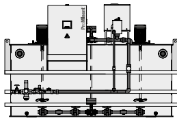
ULTROMAT ULPa pour polymères en poudre
